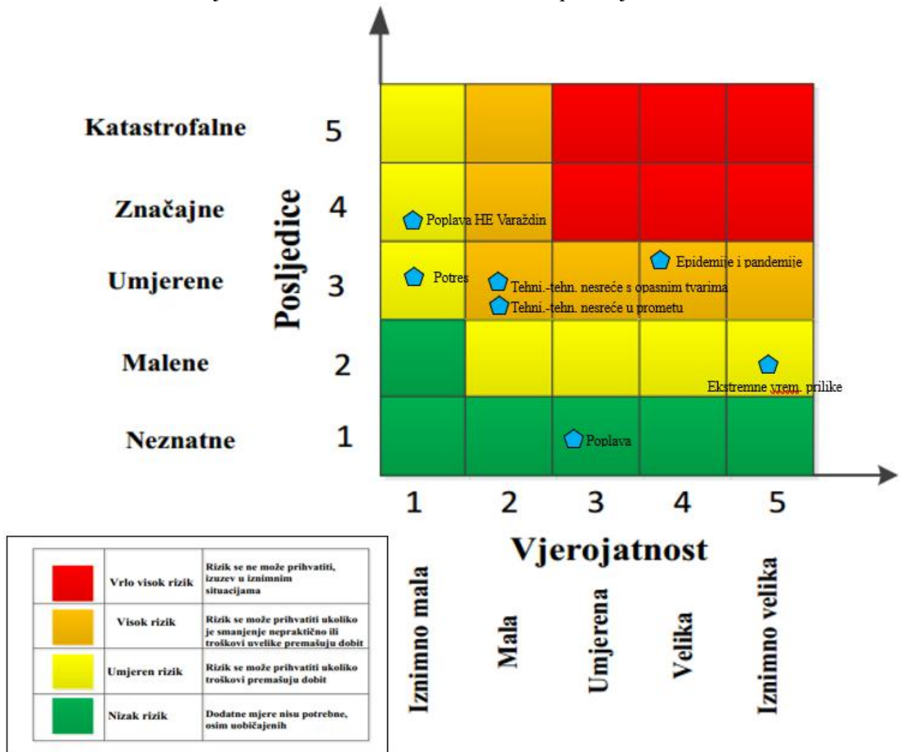
Slika 35: Zajednička matrica analiziranih rizika za područje Grada Varaždina
