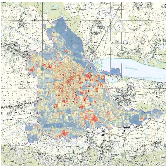
MJERLO 1:80.000 TEMPERATURNI OBILJEŽJA ZEMLJIŠTA - LIPANJ 2022. 15°C >35°C
