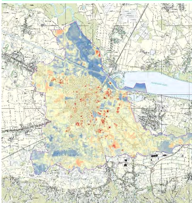
MJERLO 1:80.000 TEMPERATURNI OBILJEŽJA ZEMLJIŠTA - KOLOVOZ 2022. 15°C >35°C
