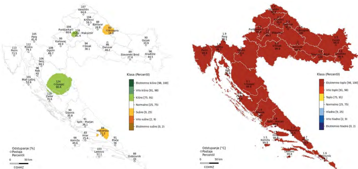
Grafički prikaz 29. Odstupanja godišnjih temp. zraka ( ^{\circ}\text{C} ) i odstupanje količine oborine (%) za 2024. godinu 122 . Izvor podataka: DHMZ, obrada autora.
