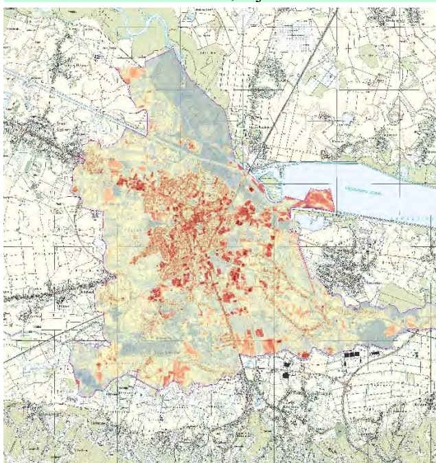
MJERLO 1:80.000 TEMPERATURNI OBILJEŽJA ZEMLJIŠTA - RUJAN 2022. 15°C >35°C
