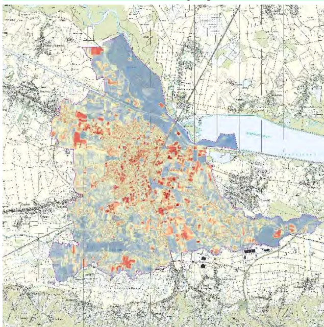
MJERLO 1:80.000 TEMPERATURNI OBILJEŽJA ZEMLJIŠTA - SRPANJ 2022. 15°C >35°C
