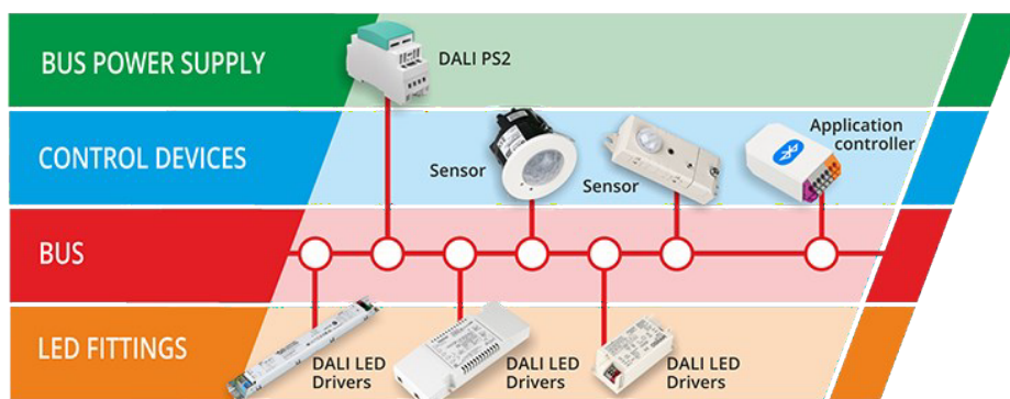
Slika 6 Inteligentni sustav upravljanja korištenjem DALI sustava iv
