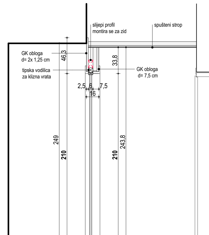
PRESJEK
