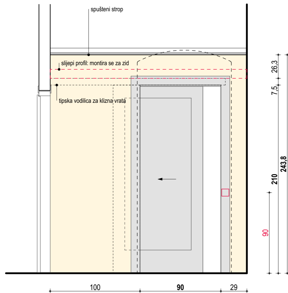
POGLED A
