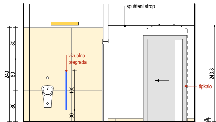
POGLED D
