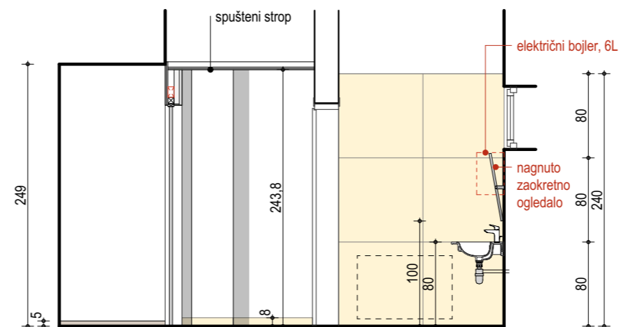
POGLED E
