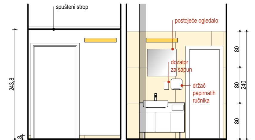
POGLED C
