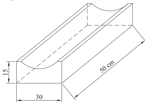
BETONSKA KANALICA (RIGOLA)
