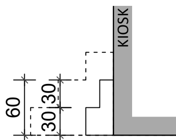
PRESJEK B-B
