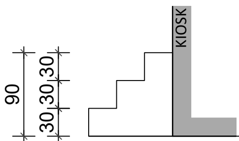
PRESJEK A-A
