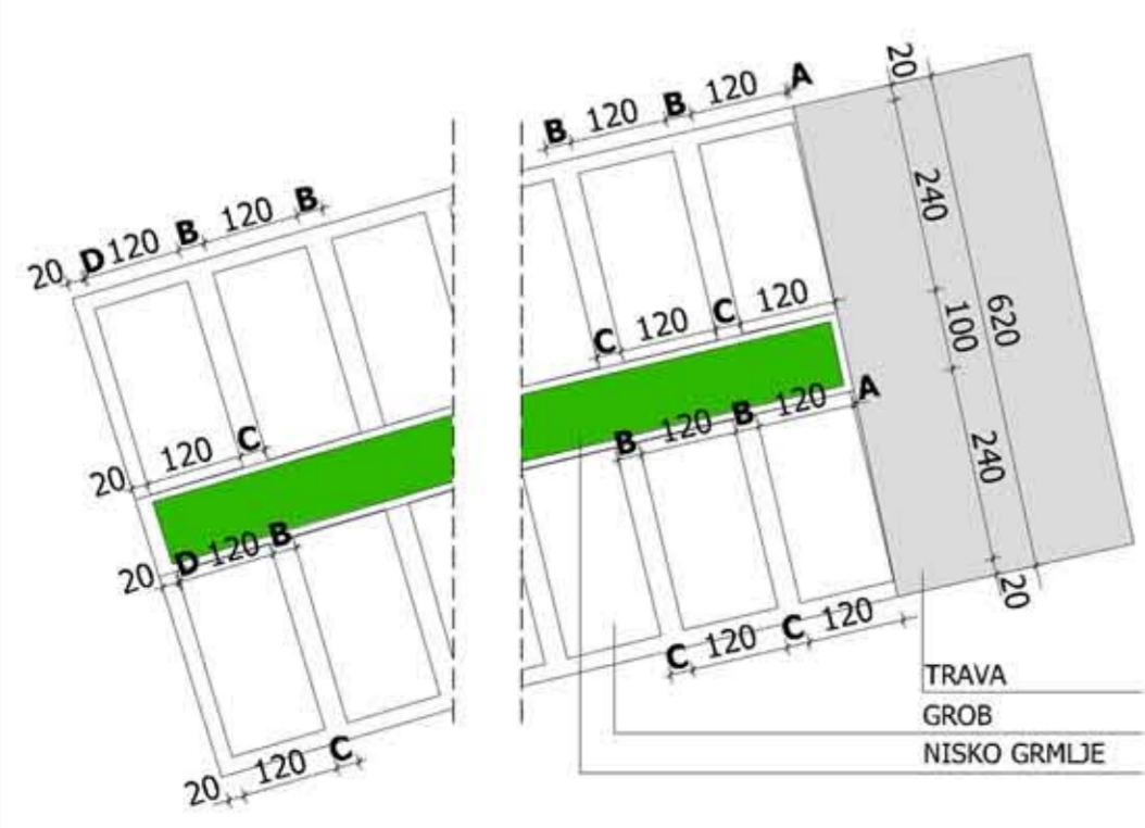
DETALJ PRIKAZA RASPOREDA UKOPNIH MJESTA U KARAKTERISTIČNOM REDU GROBNOG POLJA M. 1:100
